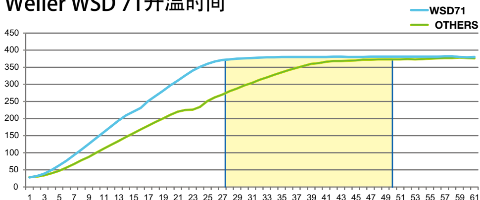
Weller WSD 71升温时间
